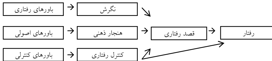
شکل 1 مدل رفتار برنامه‌ریزی شده [27]
